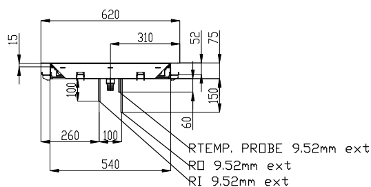
Zij aanzicht
