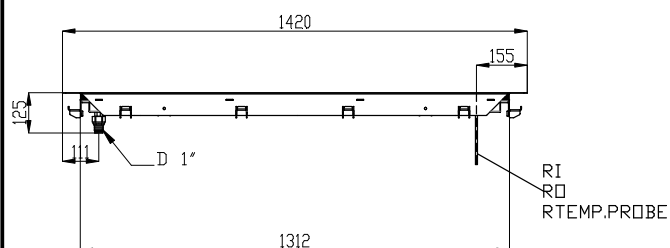
Zij aanzicht
